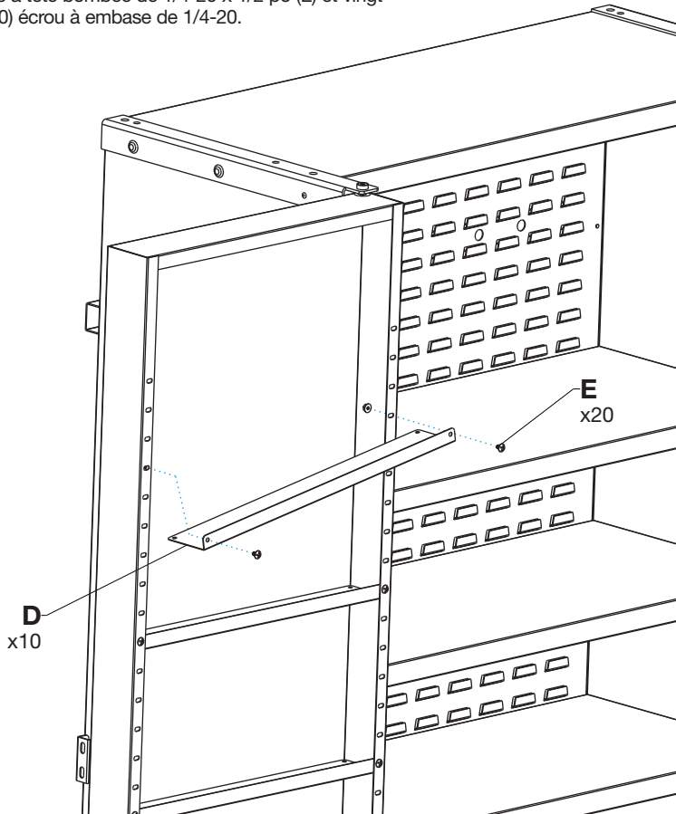
Cabinet with Shelves Only Armario con estantes solamente Armoire avec étagères seulement
